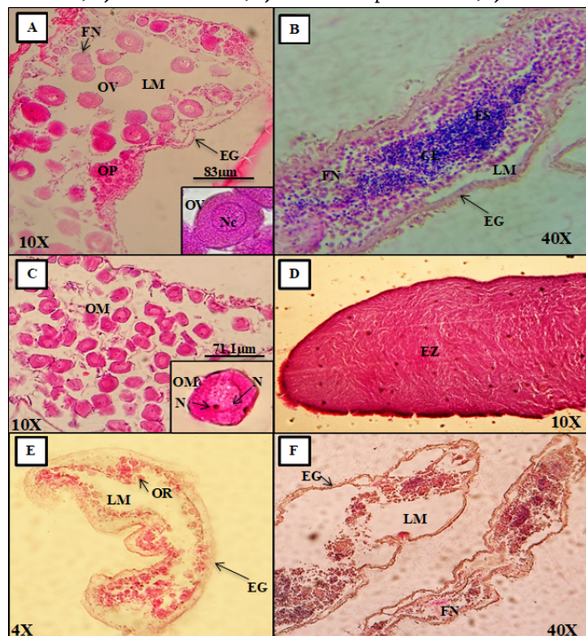
Figura 3. Estados de madurez gonadal para hembras y machos en individuos colectados de H. grisea en la bahía de Cispatá, a) Hembra en crecimiento, b) Macho en crecimiento, c) Hembra en madurez, d) Macho maduro, e) Hembra en post-desove, f) Macho
