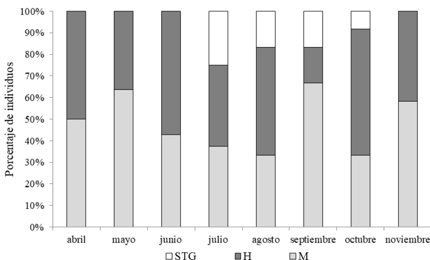
Figura 2. Porcentaje de individuos machos (M), hembras (H) y sin tejido gonadal (STG) registrados en el sector La Ahumadera, bahía de Cispatá.
