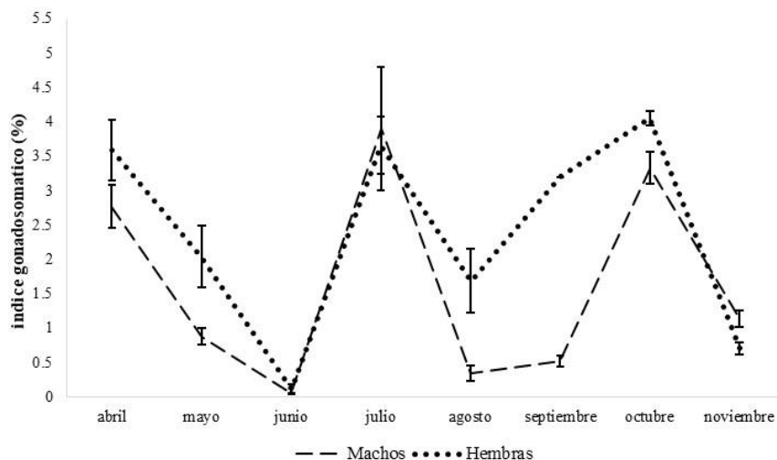
Figura 5. Promedio mensual por sexos del índice gonadosomático y sus errores estándares.
