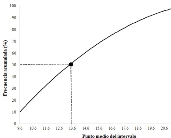
Figura 4. Probabilidad de madurez sexual con base en la longitud corporal de Holothuria grisea en la bahía de Cispatá.
